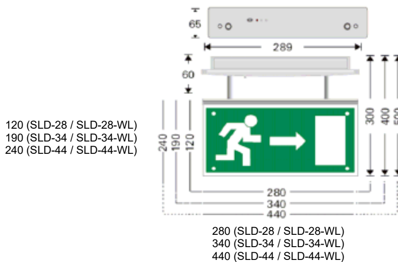
Dimensjoner (mm)
