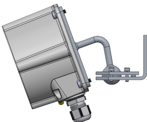
Braketten med flammedetektoren sett fra siden. Innendørs bruk
