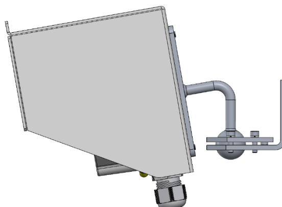
Braketten med værbraketten og flammedetektoren sett fra siden. Utendørs bruk
