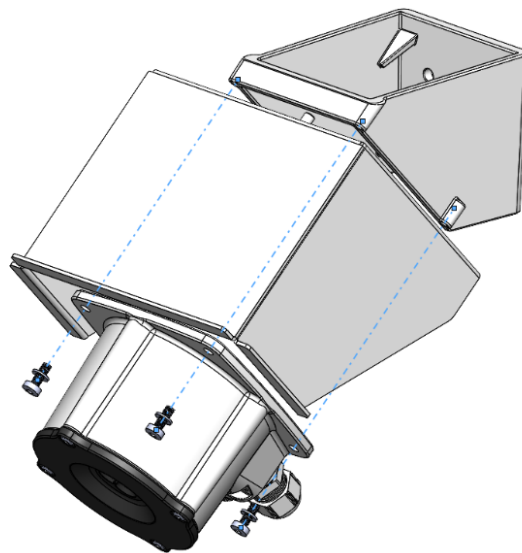
Braketten med værbraketten og flammedektoren sett fra siden. Utendørs bruk
